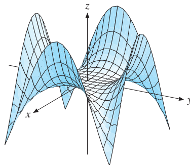
Figure 3 z = x^4 - 3x^2y^2 + y^4
